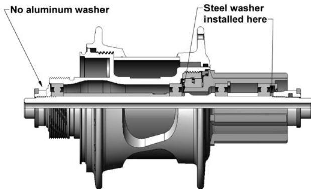
SL Hub for Campagnolo system
